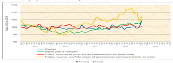
Graphique 12 — Indices de prix des matériaux de construction
